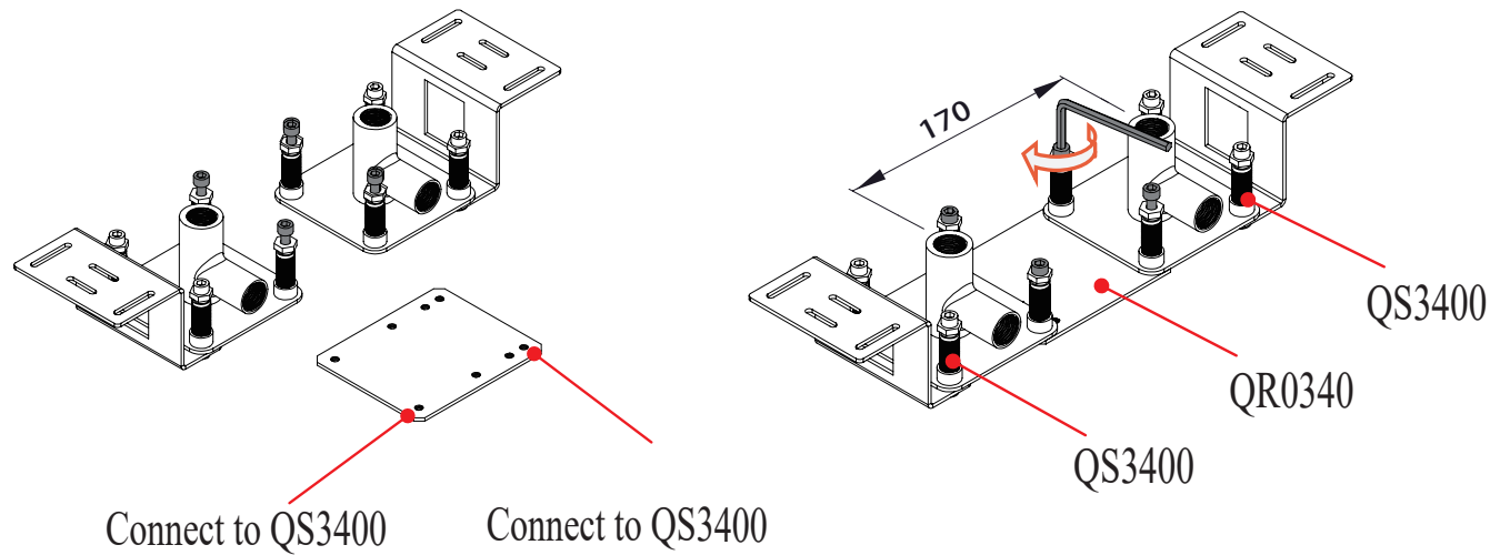
QS3400+QS3400
