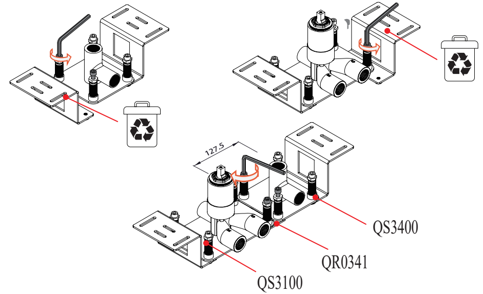
QS3400+QS3100 (Left)
