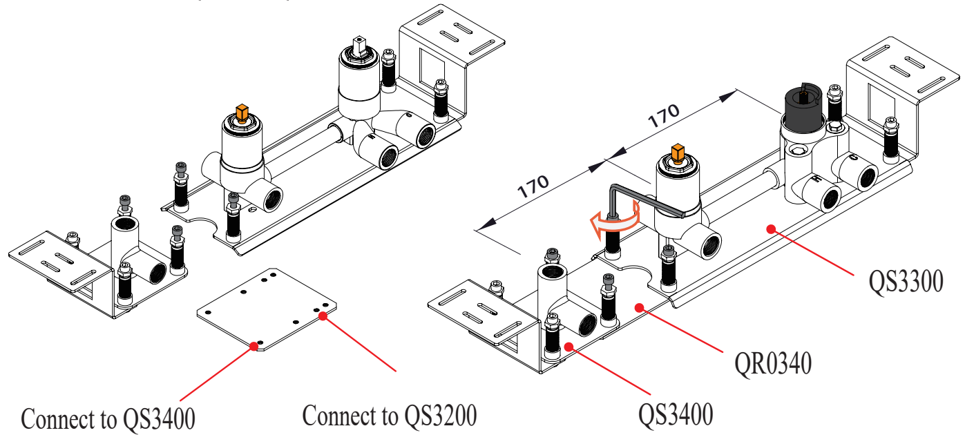
QS3400+QS3300
