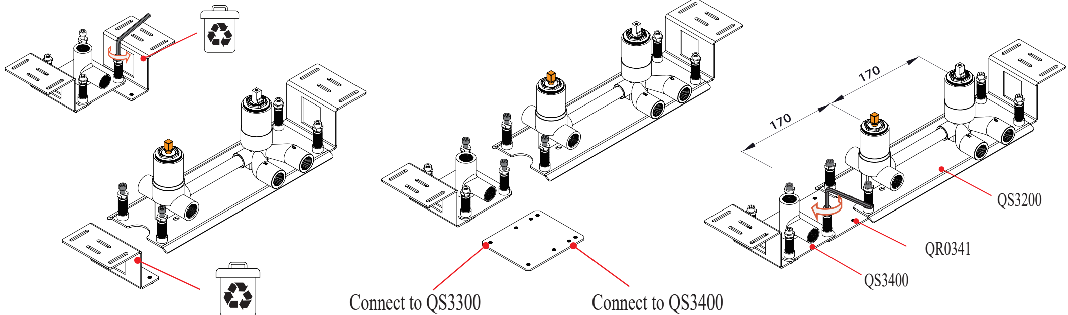
QS3400+QS3200
