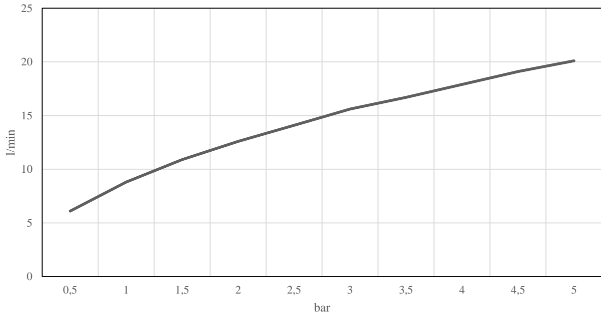
QS3200 flow rate(l/min)
